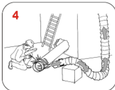
4 Aspirazione fumi di saldatura in lavori al chiuso
